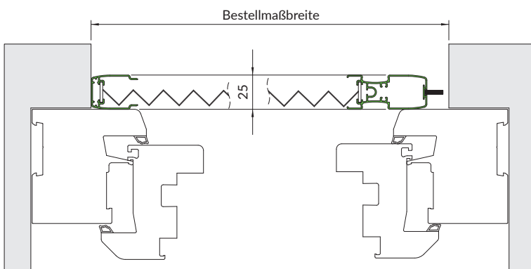
Horizontalschnitt PP 25 M 1:5
