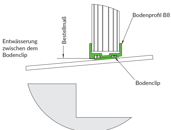
Bodendetail schräger/waagerechter Boden
