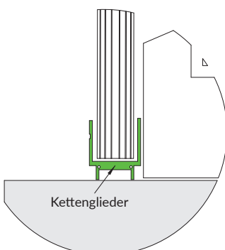
Bodendetail
