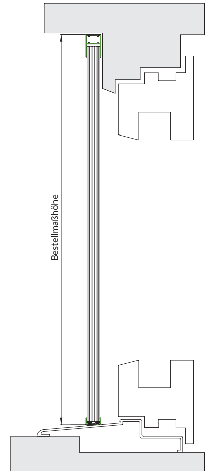
Vertikalschnitt P20-1R3 M 1:5
