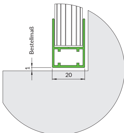
Bodendetail
