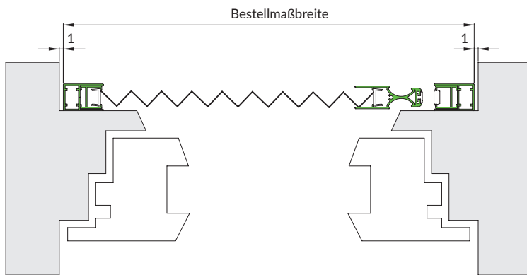
Horizontalschnitt P20-1R4 M 1:4
