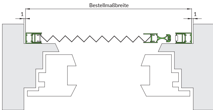
Horizontalschnitt P20-1R3 M 1:4
