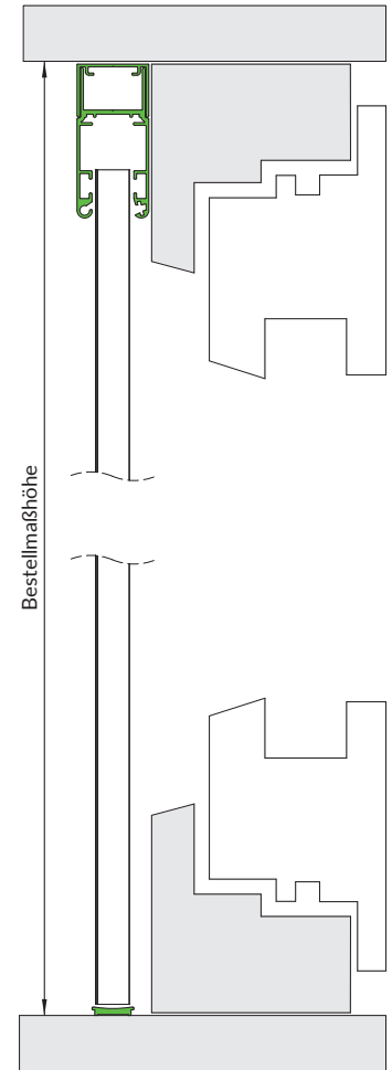
Vertikalschnitt PP 25 M 1:3
