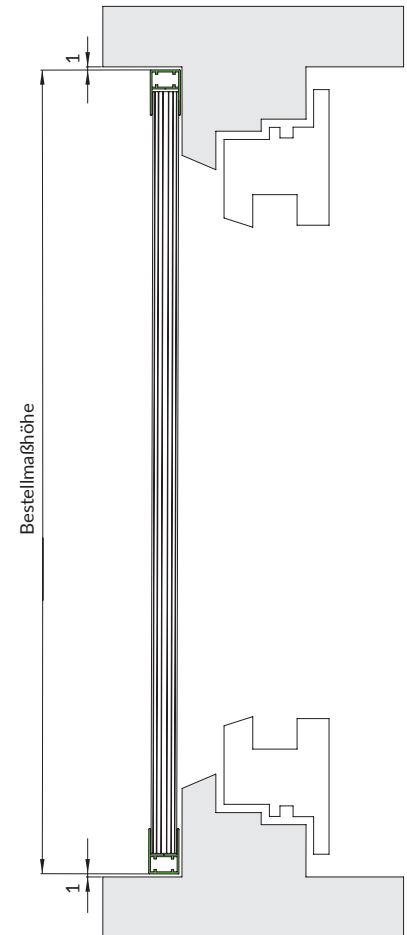
Vertikalschnitt P20-1R4 M 1:5
