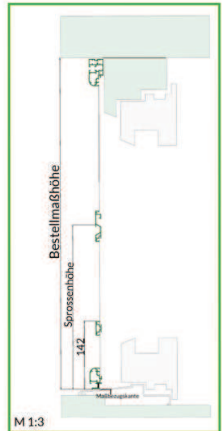
Vertikalschnitt
