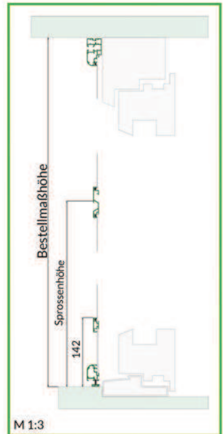
Vertikalschnitt
