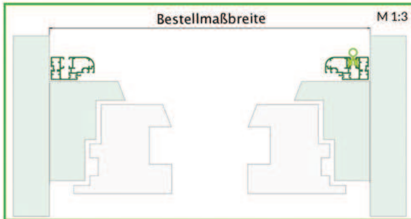
Horizontalschnitt
