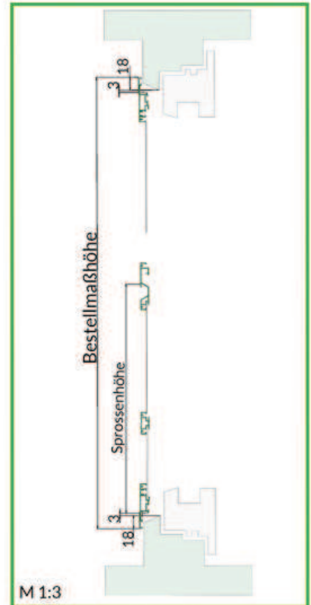
Vertikalschnitt
